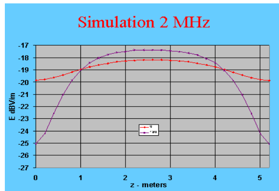
Figura 1 – Campo Elétrico no eixo “z”, em x=2.3 m e y=1 m.
